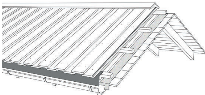
Klassiskt trätak
