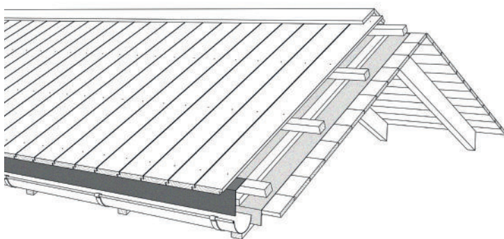
Concise trätak
